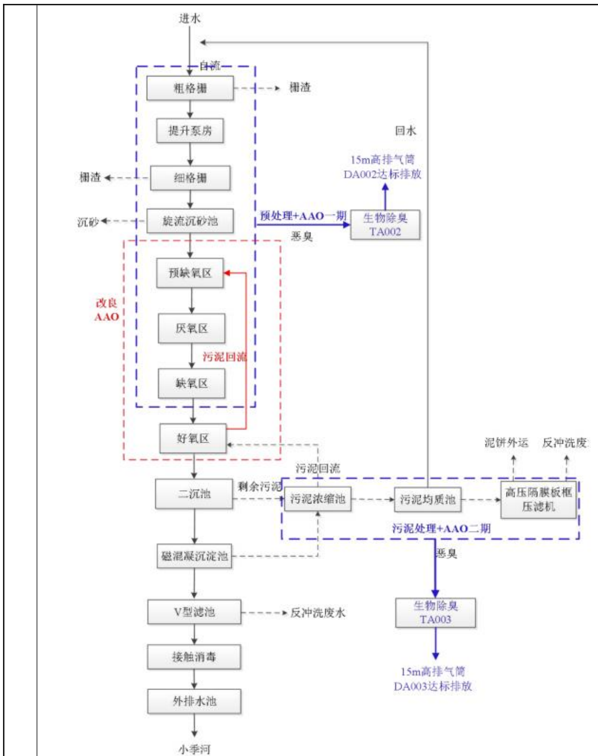
图 4-2 枣庄台儿庄区北控水务有限公司污水处理工艺流程
