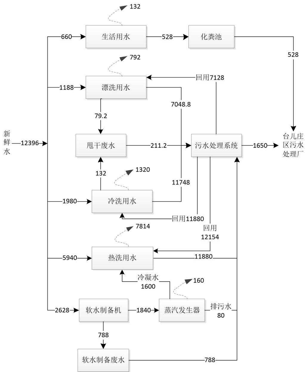
图 2-2 项目建成后全厂用水水平衡图（单位：m³/a）
