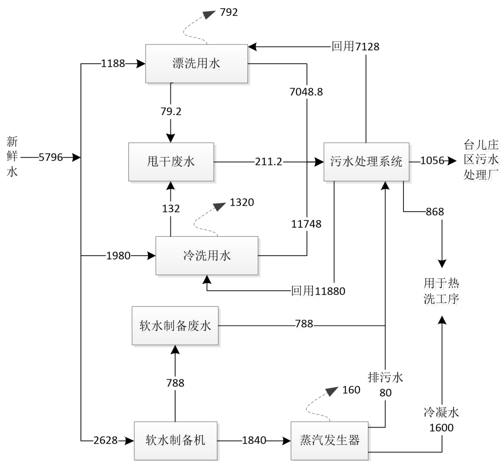
图 2-1 项目新增用水水平衡图（单位：m 3 /a）
