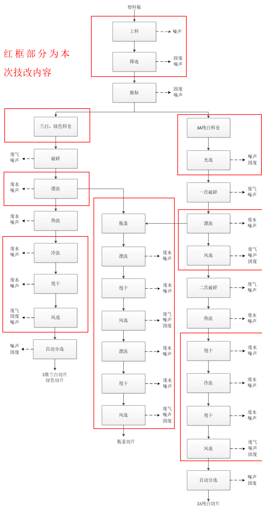
图2-2 工艺流程和产污环节分析图
