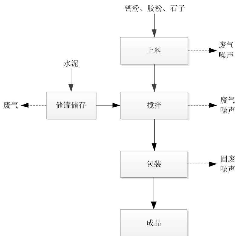
图2-3 瓷砖粘接剂、外墙腻子工艺流程和产污环节分析图
