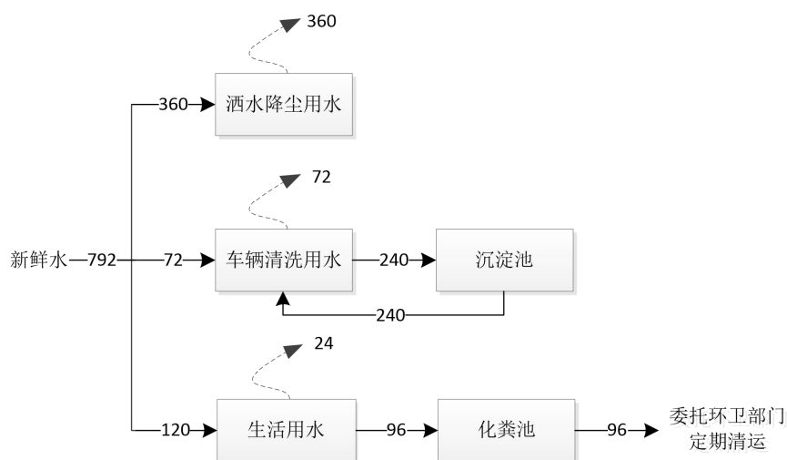
图 2-1 项目水平衡图（单位：m 3 /a）
